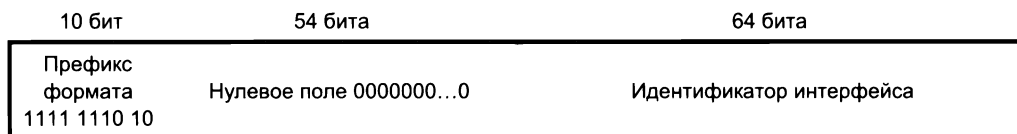
Рис. 17.3. Формат адреса уровня линии связи
