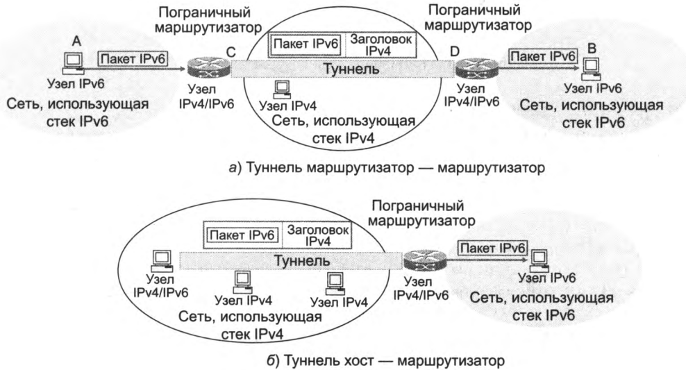
Рис. 17.18. Согласование технологий IPv4 и IPv6 путем туннелирования
