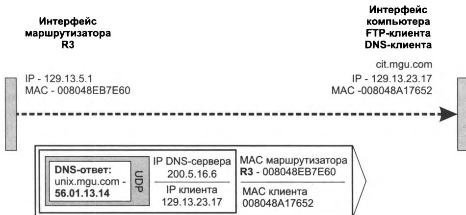
Рис. 14.8. Кадр Ethernet с DNS-ответом, отправленный с маршрутизатора R3 компьютеру-клиенту
