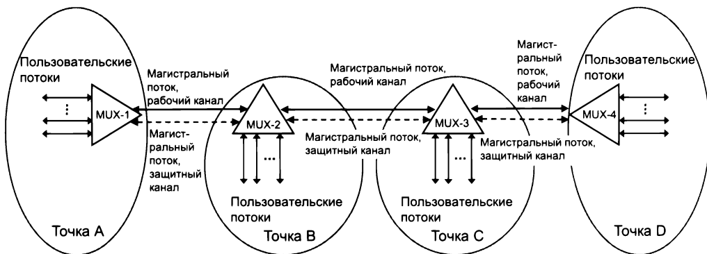
Рис. 8.19. Защита мультимплексной секции
