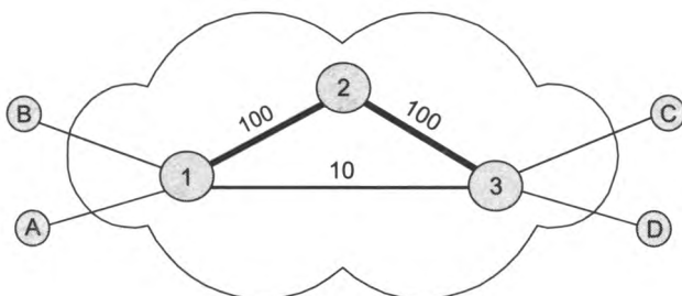
Рис. 2.13. Выбор маршрута
