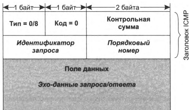
Рис. 14.17. Формат ICMP-сообщений типа эхо-запрос и эхо-ответ
