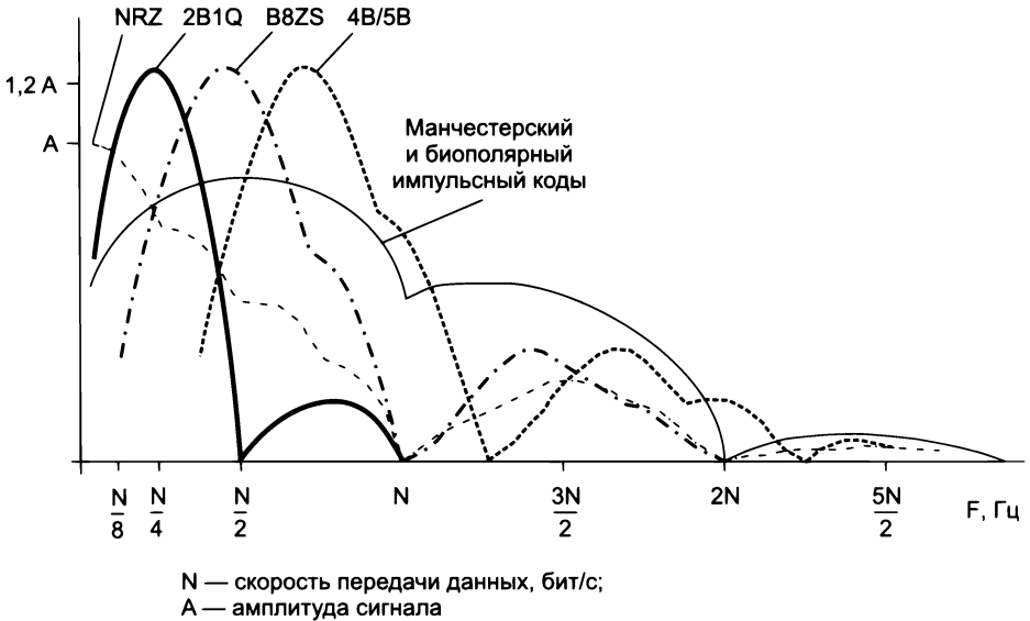
Рис. 7.6. Спектры потенциальных и импульсных кодов
