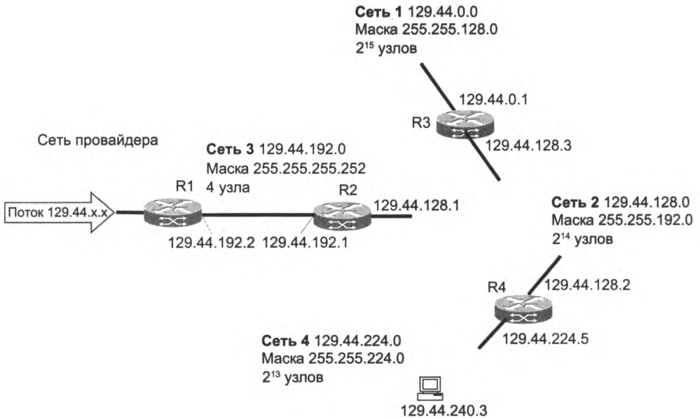
Рис. 14.12. Структуризация сети масками переменной длины
