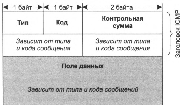
Рис. 14.14. Формат ICMP-сообщения
