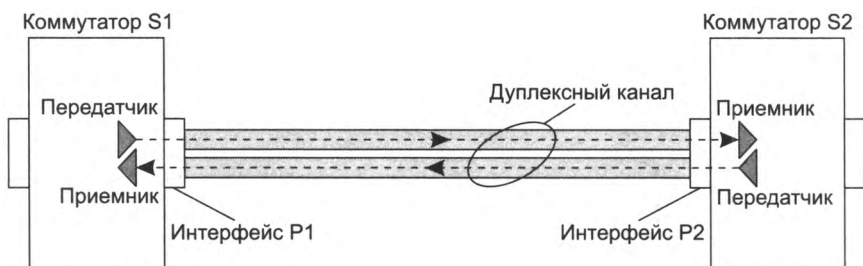
Рис. 2.18. Дуплексный канал — разделяемая среда отсутствует
