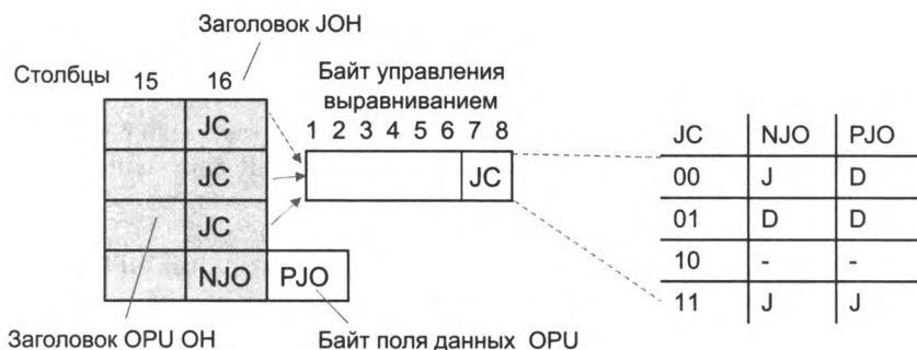
Рис. 9.12. Заголовок выравнивания JOH и байты выравнивания NJO и PJO
