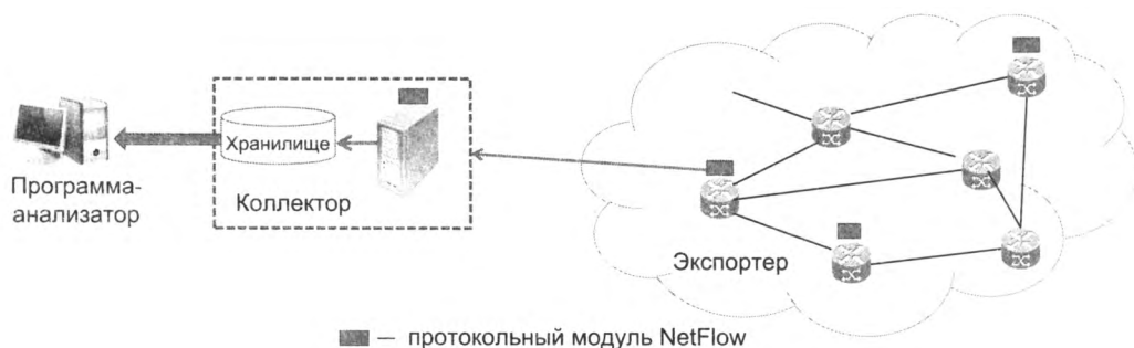
Рис. 28.10. Типичная система мониторинга на базе NetFlow
