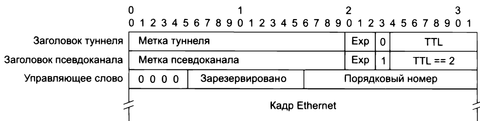
Рис. 20.23. Формат инкапсуляции Ethernet поверх MPLS
