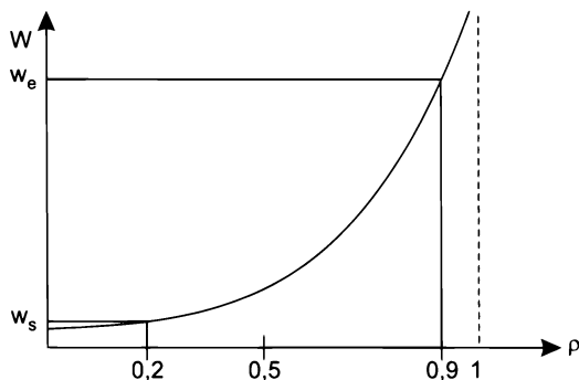
Рис. 5.13. Обслуживание эластичного и чувствительного к задержкам трафика
