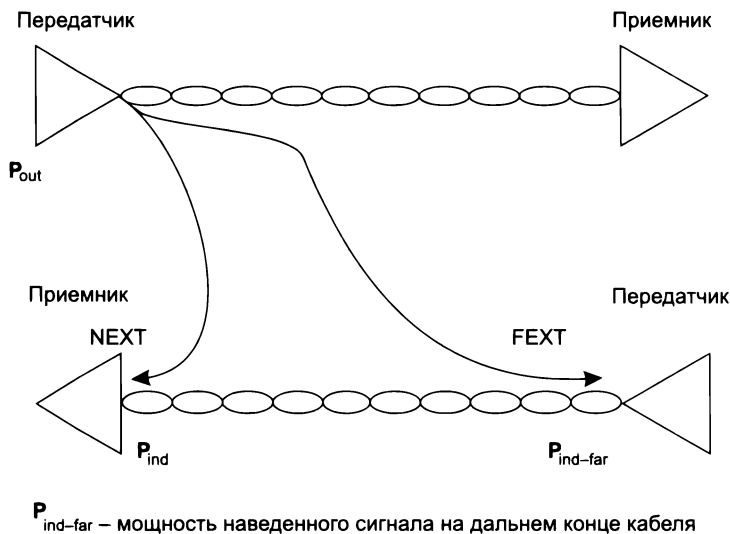
Рис. 6.17. Переходное затухание
