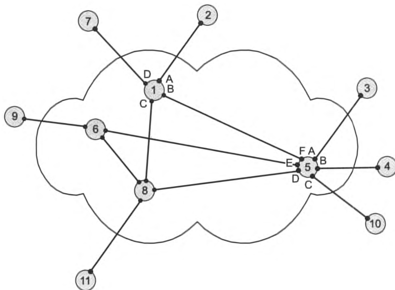
Рис. 2.15. Коммутационная сеть
