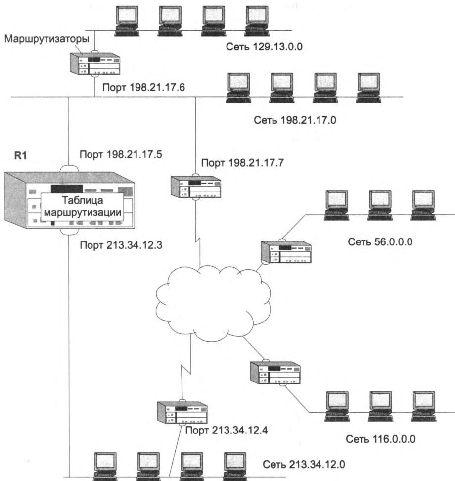
Рис. 14.3. Пример маршрутизуемой сети
