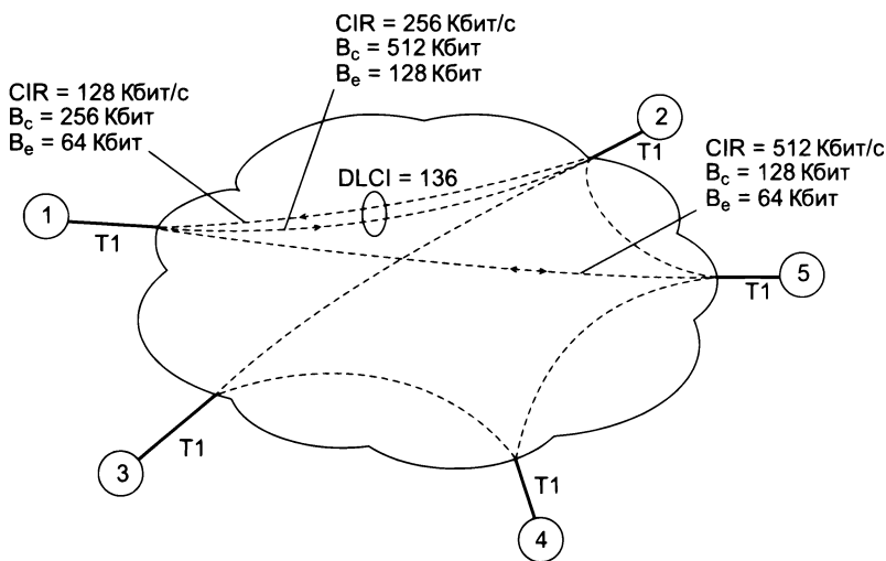
Рис. 19.4. Пример обслуживания в сети Frame Relay
