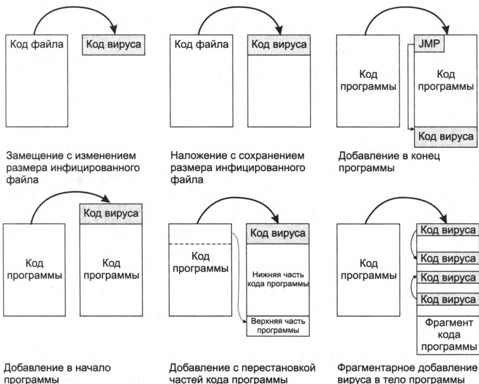
Рис. 30.3. Различные варианты расположения кода вируса в зараженных файлах
