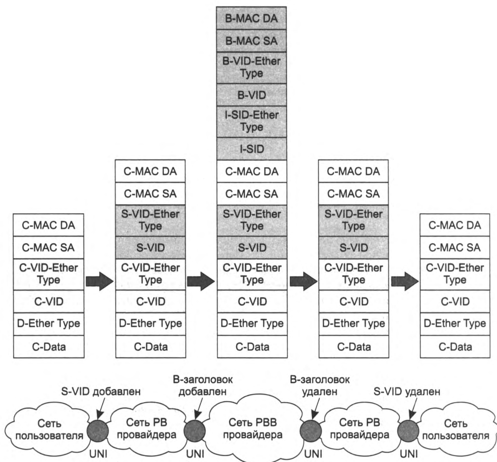
Рис. 12.5. Формат кадров при инкапсуляции MAC-in-MAC согласно стандарту IEEE 802.1ah
