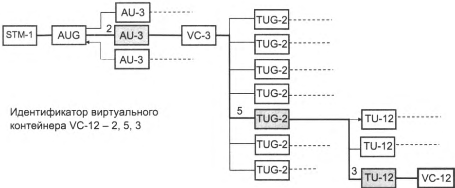
Рис. 8.17. Пример идентификации виртуального контейнера
