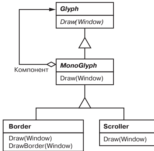
Рис. 2.7. Отношения класса MonoGlyph с другими классами
