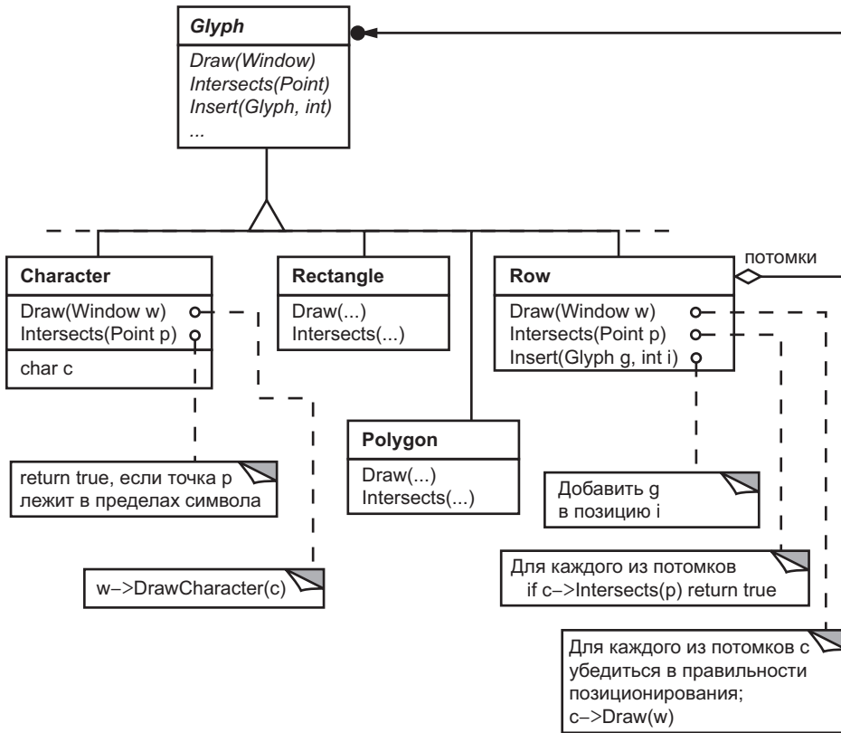
Рис. 2.4. Частичная иерархия класса Glyph
