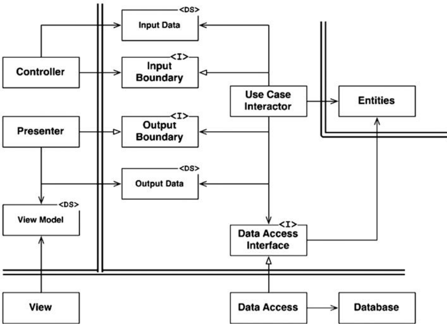
Рис. 22.2. Типичный сценарий работы веб-системы на Java, использующей базу данных
