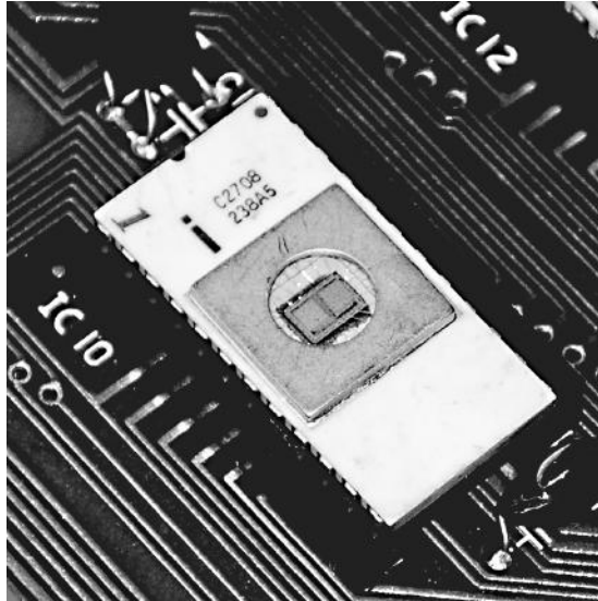
Рис. П.8. Микросхема СПЗУ (EPROM)
