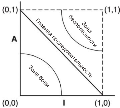
Рис. 14.13. Зоны исключения
