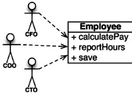
Рис. 7.1. Класс Employee
