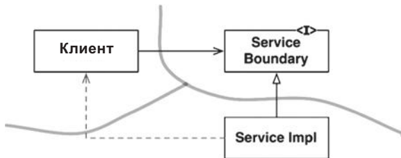
Рис. 24.1. Шаблон «Стратегия»
