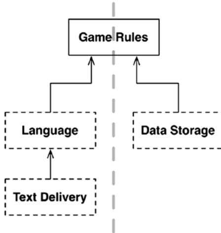
Рис. 25.4. Упрощенная диаграмма
