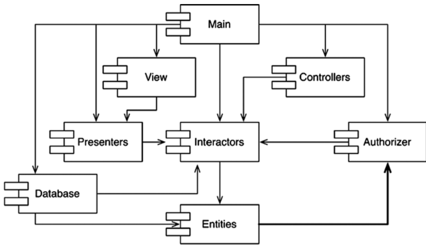
Рис. 14.2. Циклическая зависимость
