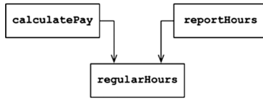
Рис. 7.2. Общий алгоритм
